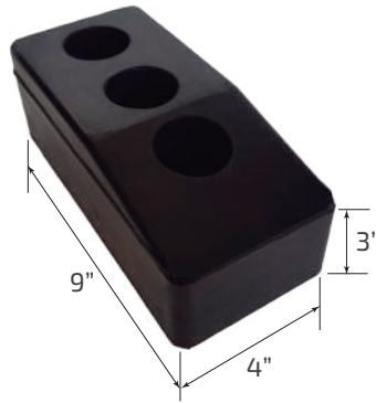
Tope EP-12 (3 orificios) H07-21
